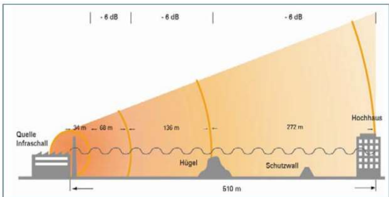
Abb. 4: Bei Infraschall ist die Wellenlänge größer als Wohnhäuser, Bäume und Schutzwälle hoch sind. Deshalb dämpfen sie ihn kaum, der Schallpegel sinkt unabhängig von der Umgebung: verdoppelt sich die Entfernung, nimmt er um sechs Dezibel ab. Im Beispiel dargestellt ist Infraschall von zehn Hertz; er hat eine Wellenlänge von 34 Metern.
